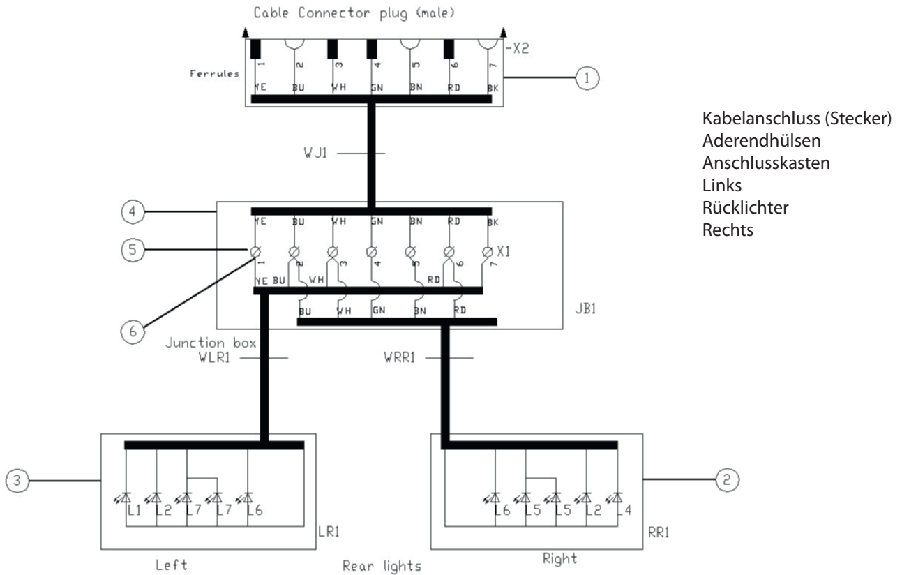
Schaltplan Rücklichter
